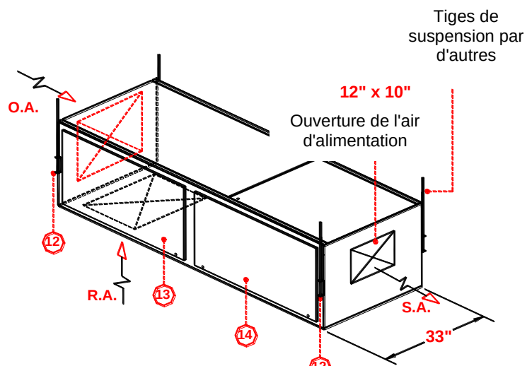
VUE ISOMÉTRIQUE (illustrée avec le panneau d'accès latéral gauche)
